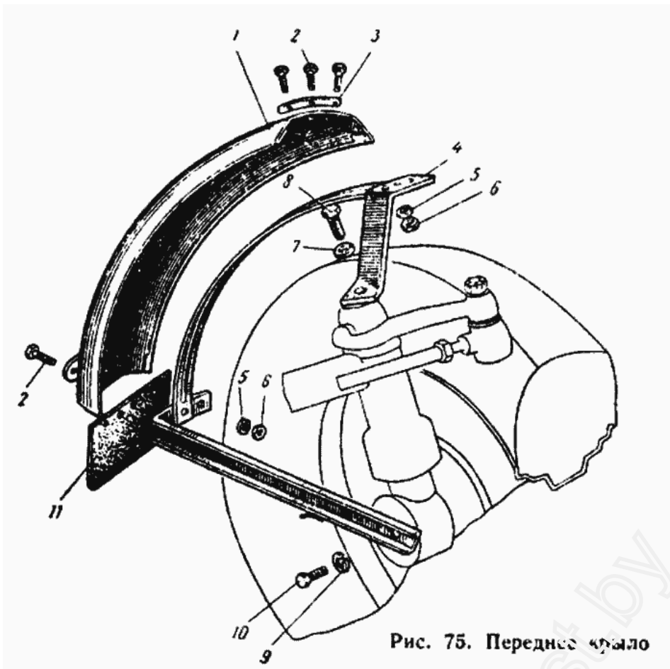
ЮМЗ-6Л Рис. 75. Переднее крыло.
