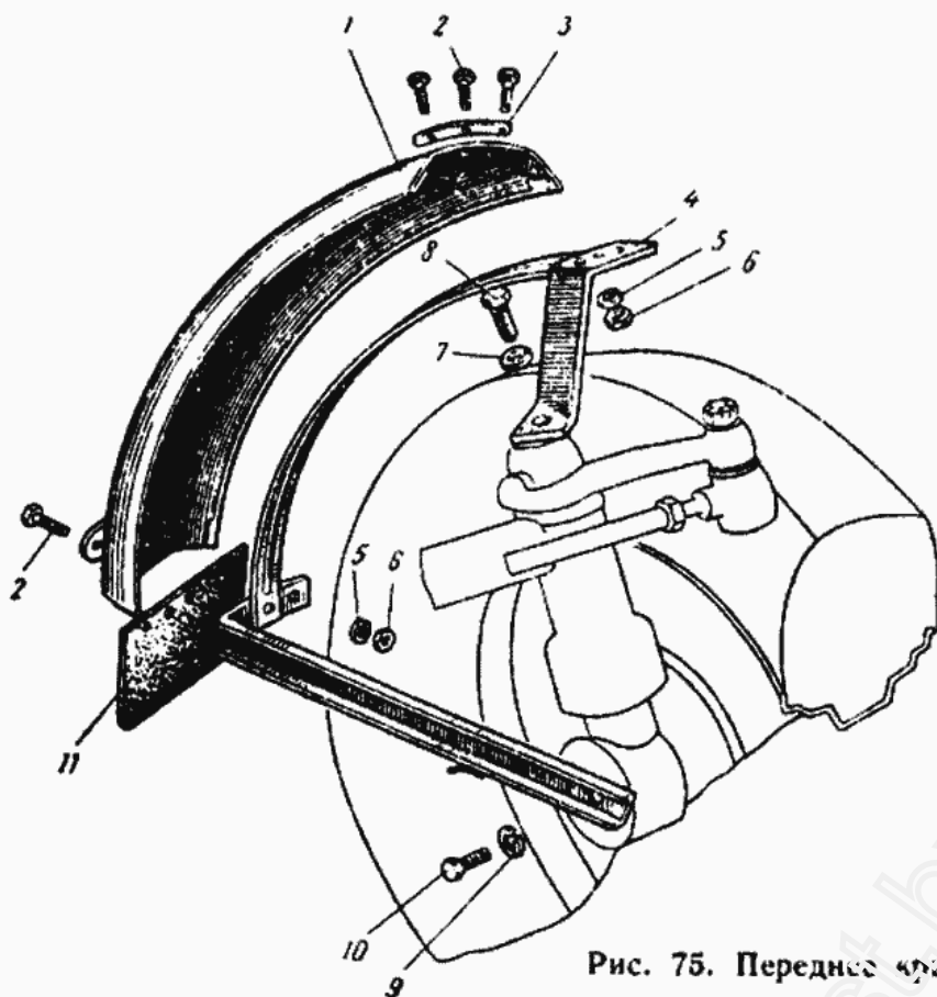
ЮМЗ-6Л Рис. 75. Переднее крыло.
